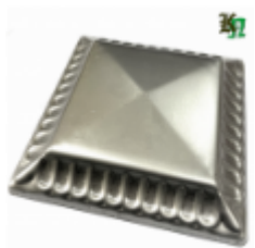
Основание балясины штампованное, арт. 8.880 170x170x1 Вес: 0.27 кг Цена: 135 руб.
