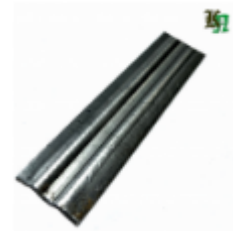
Обжимка, арт. 1509 1300х23х1,5мм Вес: 0.3 кг Цена (за штуку): 110 руб.
