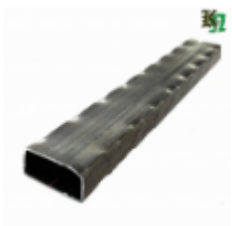
Труба профильная, арт. 40202Т 3000x40x20мм Вес: 3.9 кг Цена (за штуку): 520 руб.
