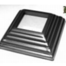
Основание блясины, арт. 13.350.01 100x100x1мм, кв.50x50мм Вес: 0.064 кг Цена: 37 руб.
