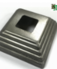
Основание баясины, арт. R10436.02 80x80x1мм, кв.25x25мм Вес: 0.075 кг Цена (за шт): 10 руб.
