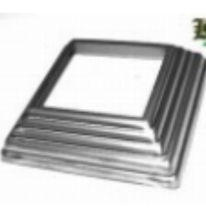
Основание блясины, арт. 13.380.01 122x122x1мм, кв.80x80мм Вес: 0.11 кг Цена: 50 руб.
