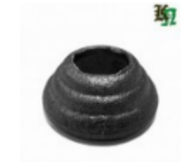
Основание баясины, арт. 7.348 д=40мм, отв.д=16мм Вес: 0.05 кг Цена: 52 руб.
